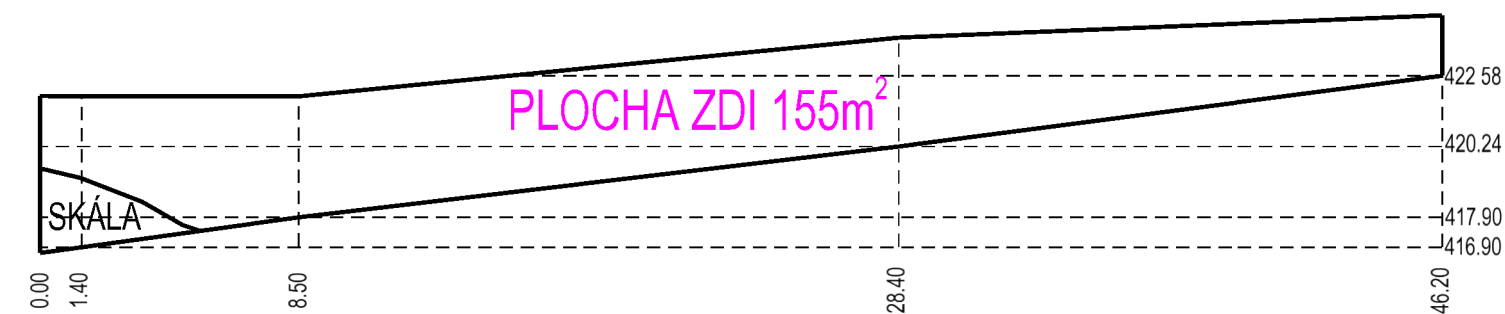
PODÉLNÝ PROFIL OPĚRNÉ ZDI
